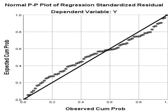
Gambar 2. Hasil Uji Normalitas P-Plot
